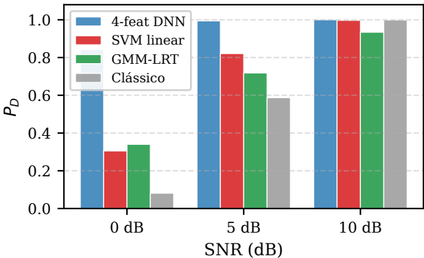
P_D em baixo SNR — \alpha = 10^{-7}
